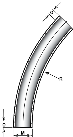
45° X 12"
